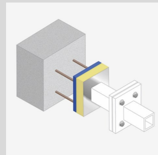
Stahl-Beton-Verbindung
